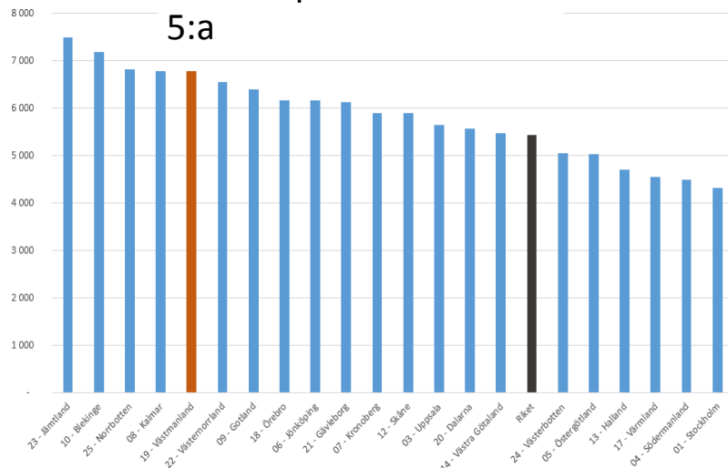
Opioider N02A
